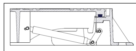
Varianta s plynovou vzpěrou
