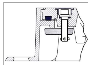
Varianta s osazením obrtlíku
