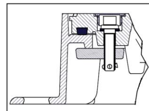
Varianta s osazením obrtlíku
